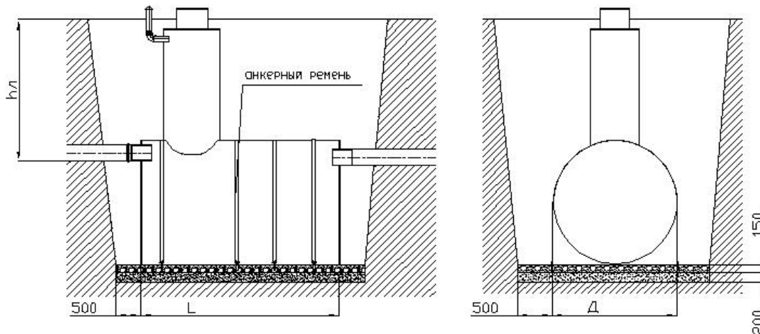
Рис 3. Устройство котлована маслобензоотделителя
