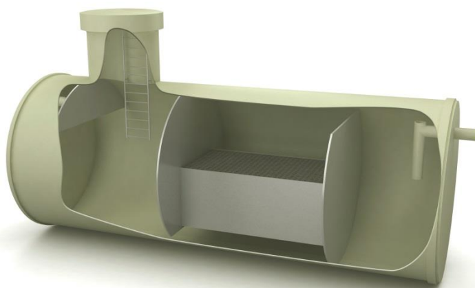
Рис 1. Внешний вид и устройство системы без сорбционного фильтра
