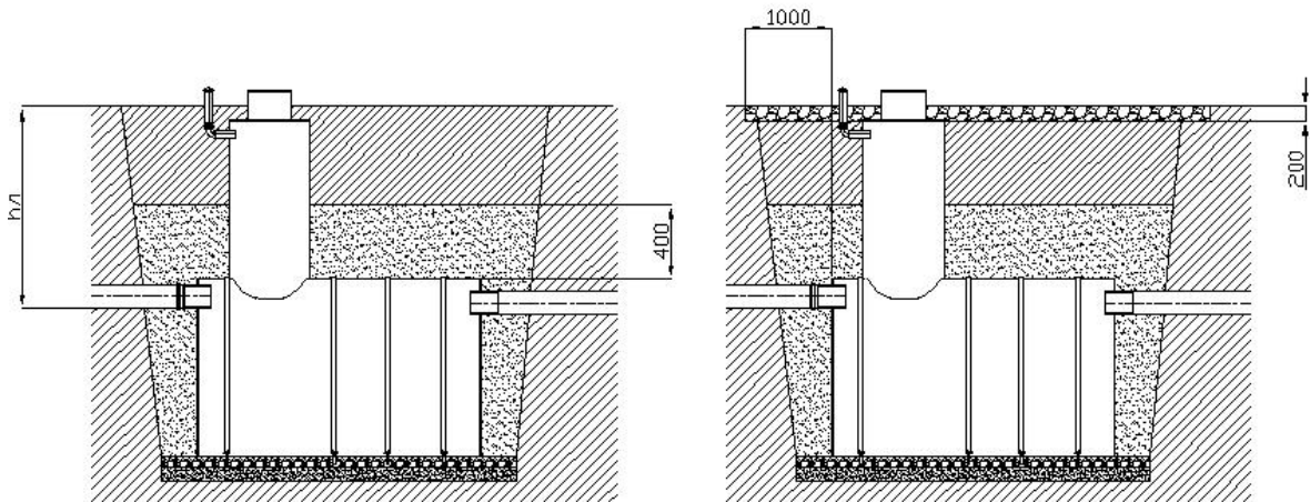
Рис 4. Обратная засыпка маслобензоотделителя
